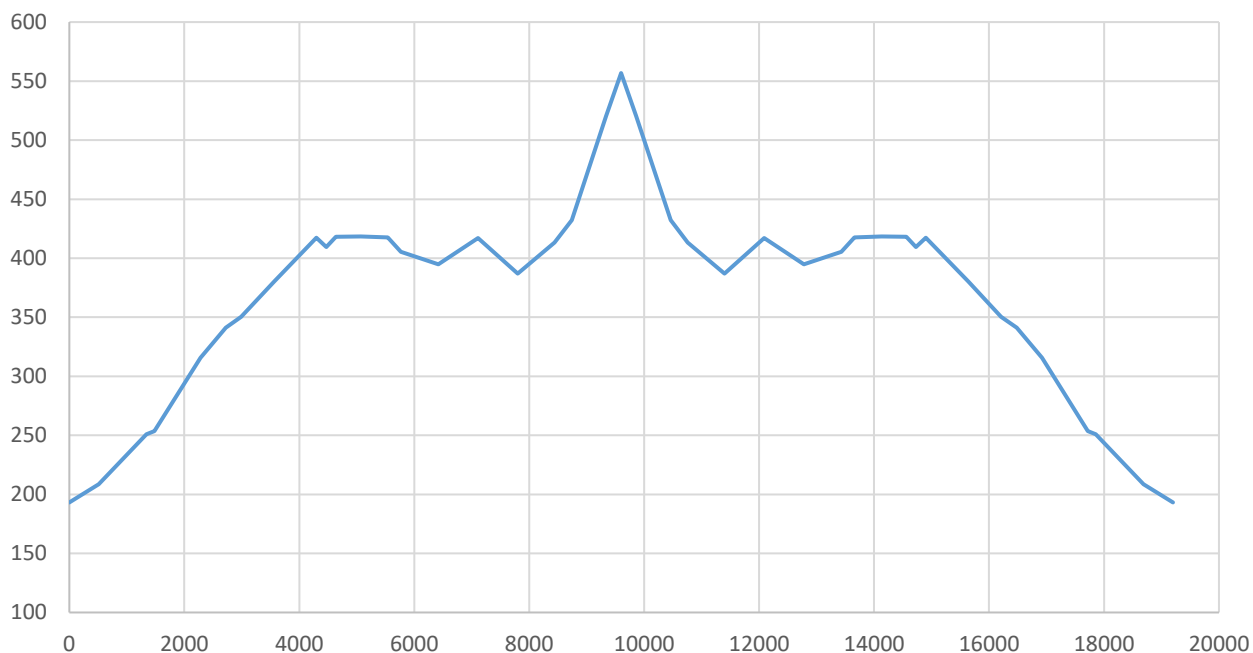
Višinski in načrtni profil Tolmin-Javorca-Tolmin
