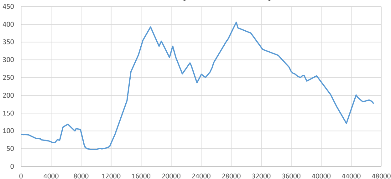
Višinski in načrtni profil Nova Gorica-Cerje-Komen-Mavhinje
