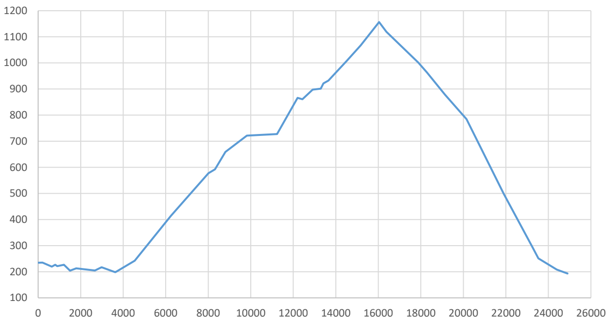
Višinski in načrtni profil Kobarid-Mrzli-Tolmin
