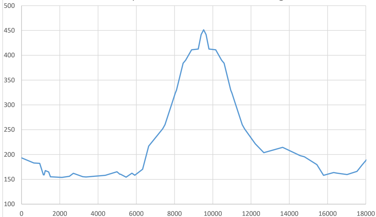
Profilo plani altimetrico Anello del Mengore
