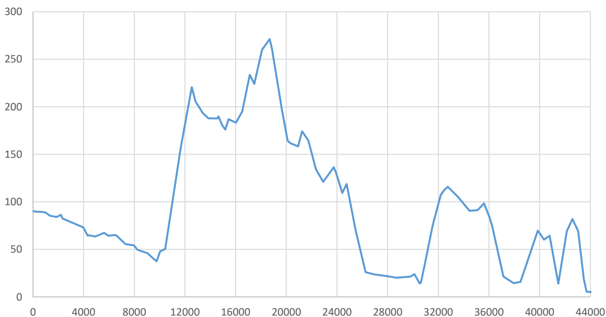
Profilo plani-altimetrico Gorizia-M. S. Michele-Monfalcone
