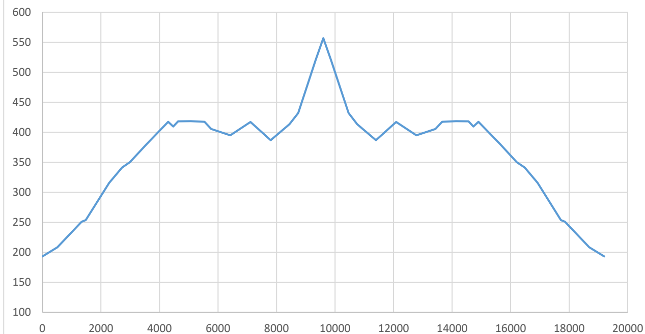
Profilo plani-altimetrico Tolmin-Javorca-Tolmin
