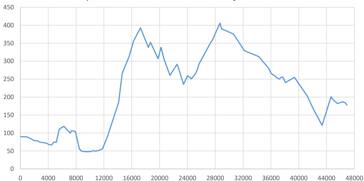
Profilo piani-altimetrico Nova Gorica-Cerje-Komen-Malchina
