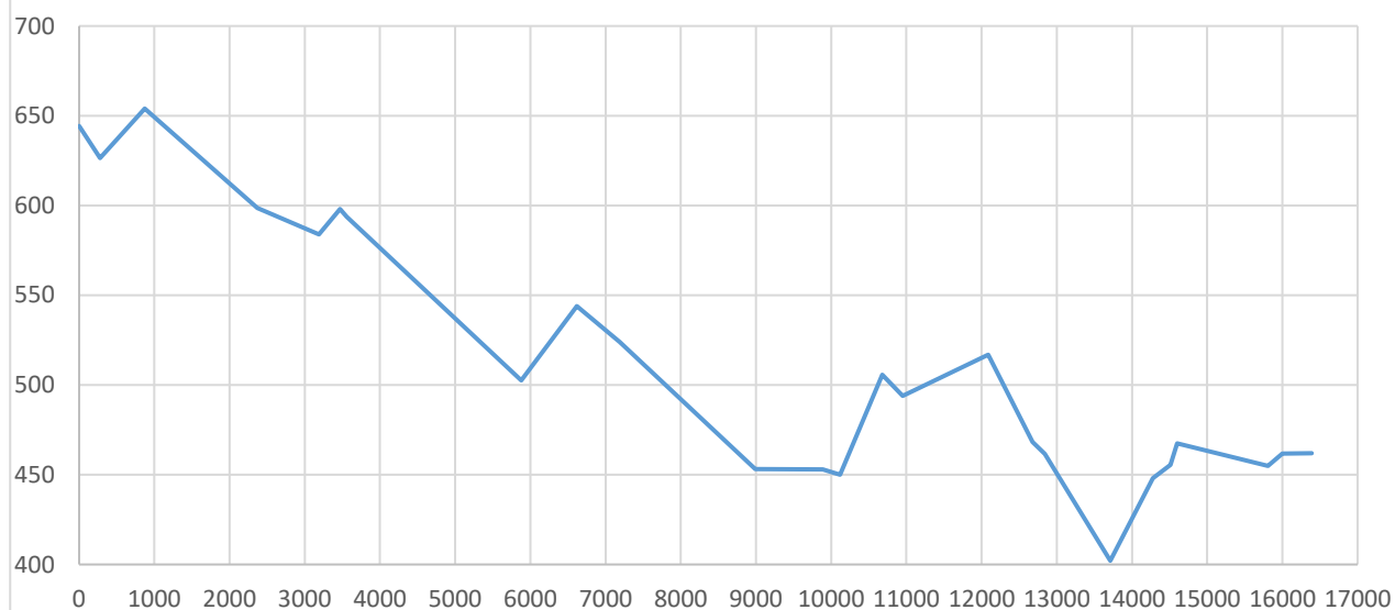
profilo piani-altimetrico tratto Stolz-Bovec
