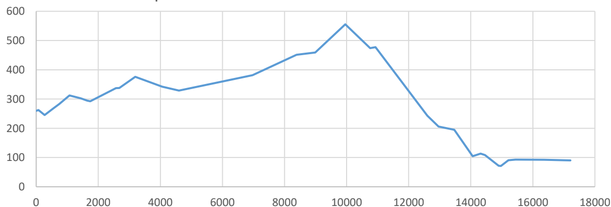
Profilo plani-altimetrico Šmartno-Sabotin-Nova Gorica
