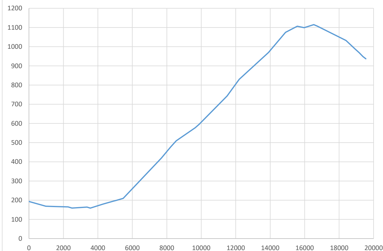
Profilo plani-altimetrico Tolmin-Kolovrat-Rif. Solarie
